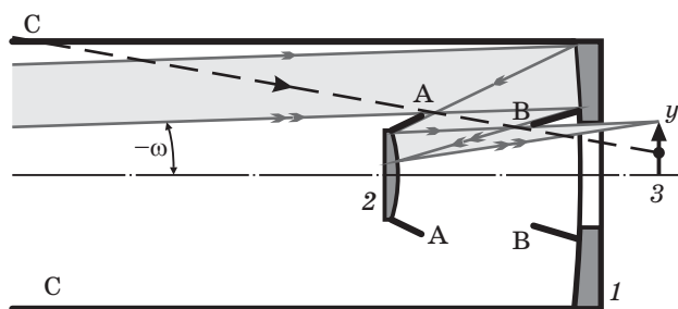
Рис. 2. Двухзеркальная система Ричи–Кретьена с защитными блендами. 1 – первое зеркало, 2 – второе зеркало, 3 – плоскость изображения.
