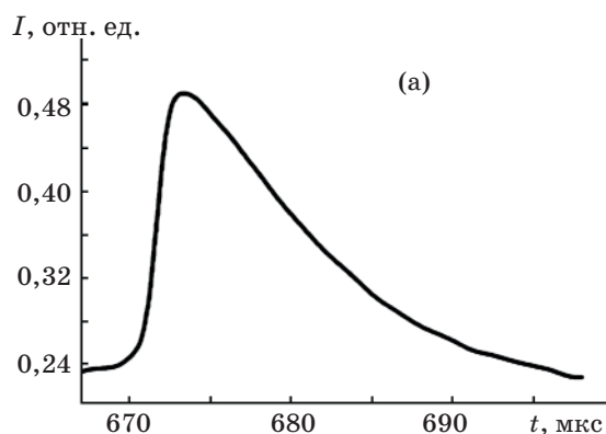
Форма вспышки МЛ органического (а) и силикатного (б) стекол после удара по поверхности стальным бойком.
