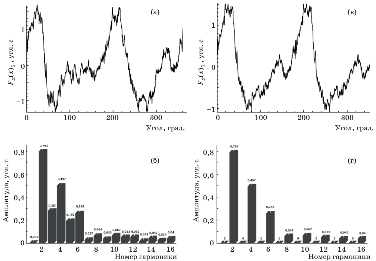
Рис. 1. Угловые погрешности F_d(x)_1 и спектральный состав угловых погрешностей для первой подложки (пояснения в тексте).
