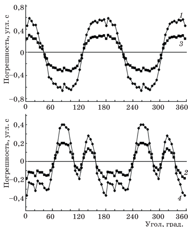
Рис. 5. Результат вычитания F_d(x)_1 - F_d(x)_2 для первой (1) и второй (2) подложек и зависимости F(x) = A_{1,2}\sin(2x + B_{1,2}) + A_{1,6}\sin(6x + B_{1,6}) для первой (3) и второй (4) подложек.
