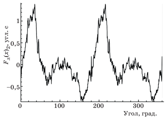
Рис. 2. Угловая погрешность расположения диаметров осей штрихов F_d(x)_2 для первой подложки.
