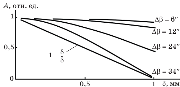
Рис. 1. Графики функции A(\Delta\beta/\delta\hat{\delta}) = J_1(4\pi\sigma_0 r \delta \Delta\beta/\hat{\delta}) / (4\pi\sigma_0 r \delta \Delta\beta/\hat{\delta}) при \Delta\beta = \text{const} и треугольной функции первой степени 1 - \delta/\hat{\delta} .
