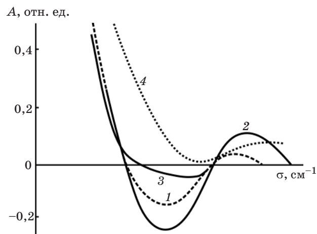
Рис. 2. АФ сканирующего двухлучевого интерферометра с параллелограммной направляющей. 1 — измеренная (спектр излучения He-Ne-лазера на \lambda = 3,39 \text{ мкм} ), 2 — вычисленная по формуле из [4], 3 — вычисленная по уравнению с аппаратной аподизацией A = J_1(4\pi\sigma_0 r \delta \Delta\beta/\hat{\delta}) / (4\pi\sigma_0 r \delta \Delta\beta/\hat{\delta}) , 4 — АФ с треугольной аподизацией первой степени 1 - \delta/\hat{\delta} .
